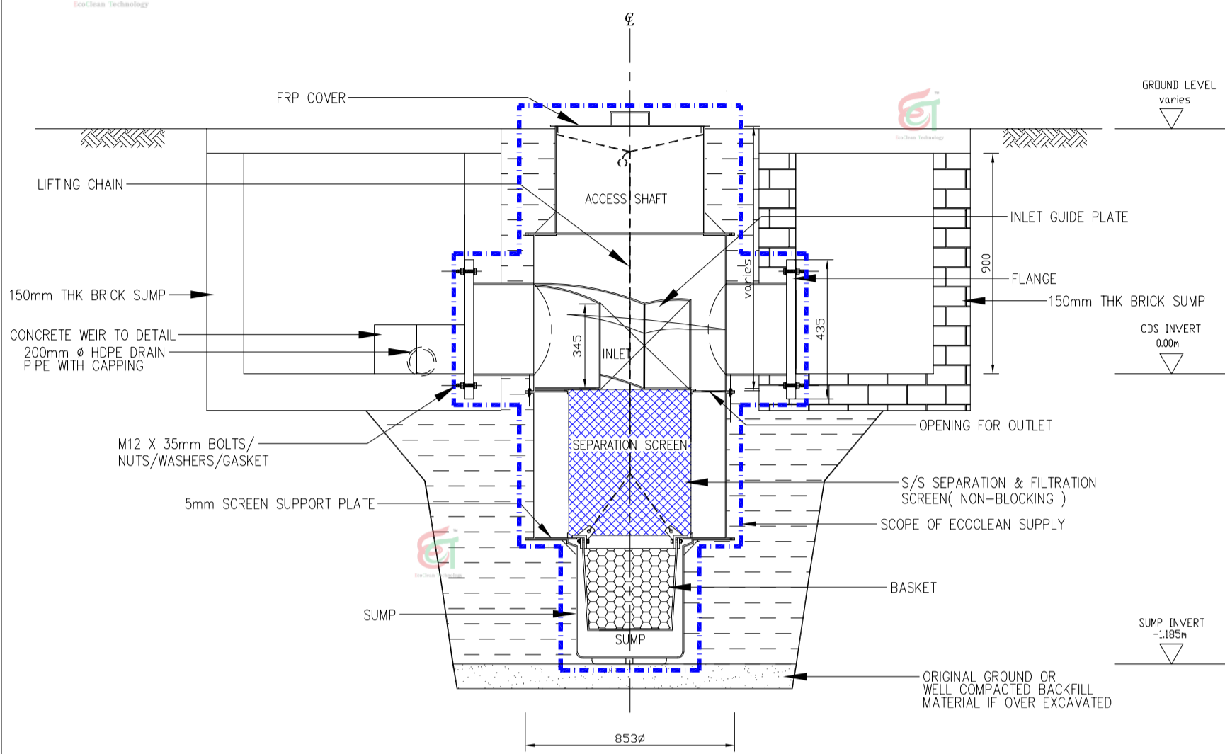
SECTION A-A
