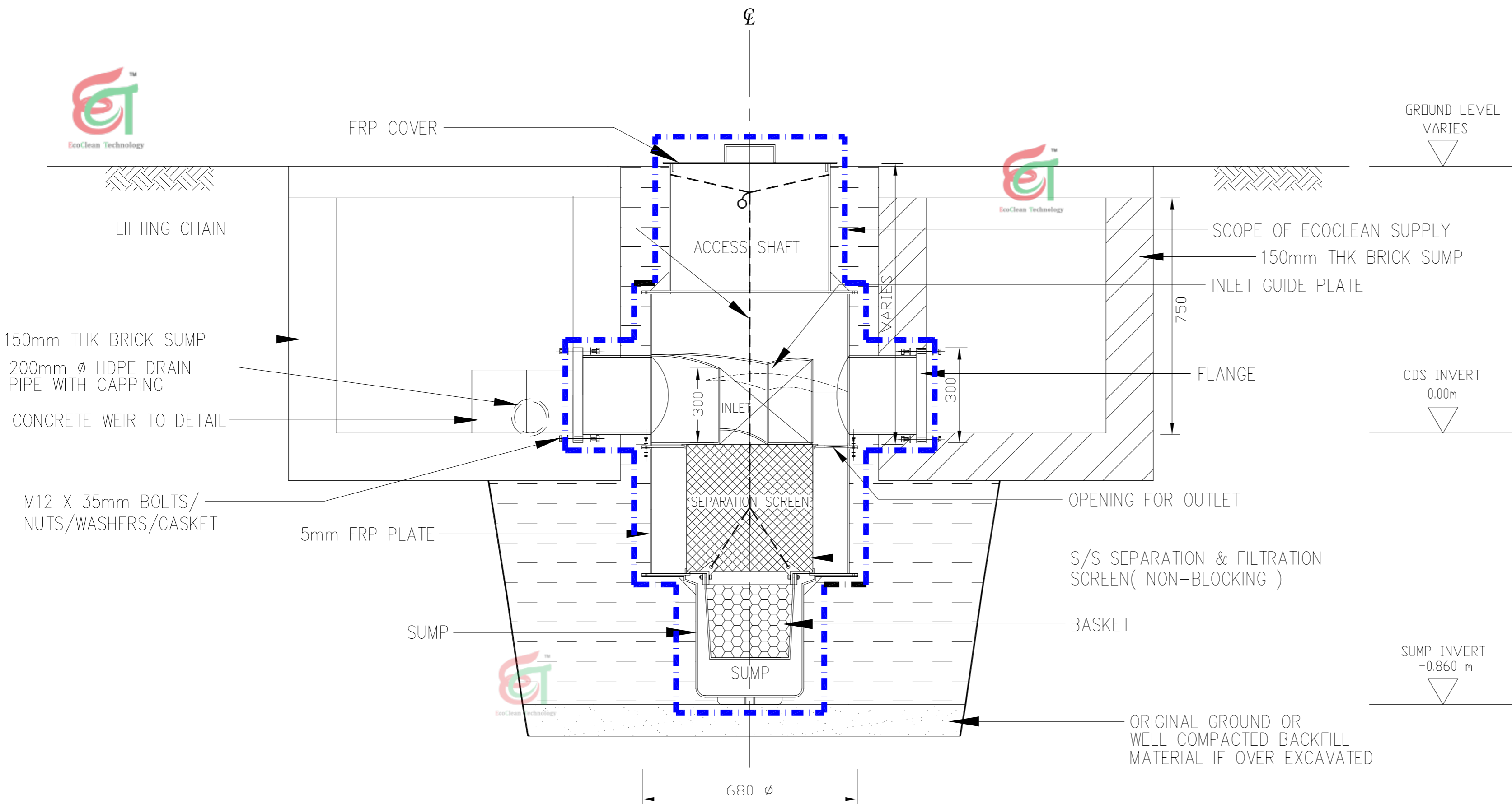
SECTION A-A
