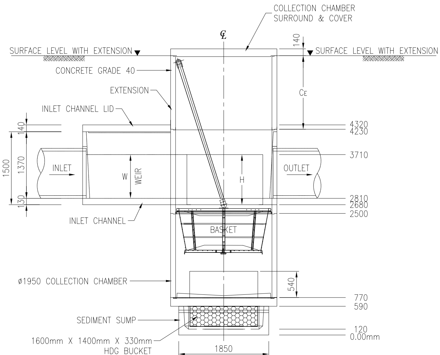
SECTION A-A
