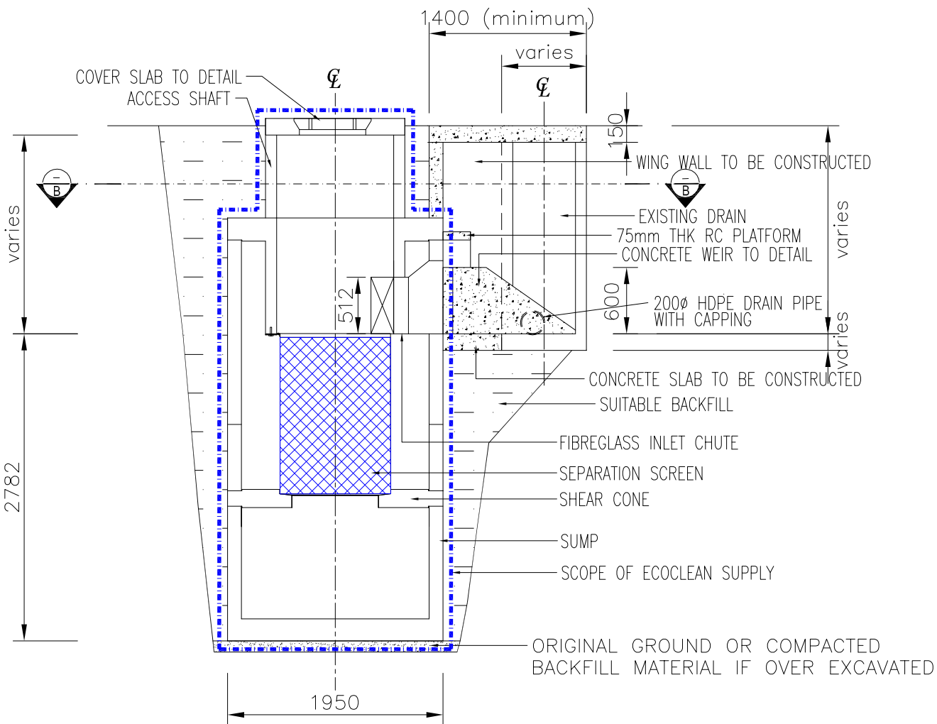
SECTION A-A
