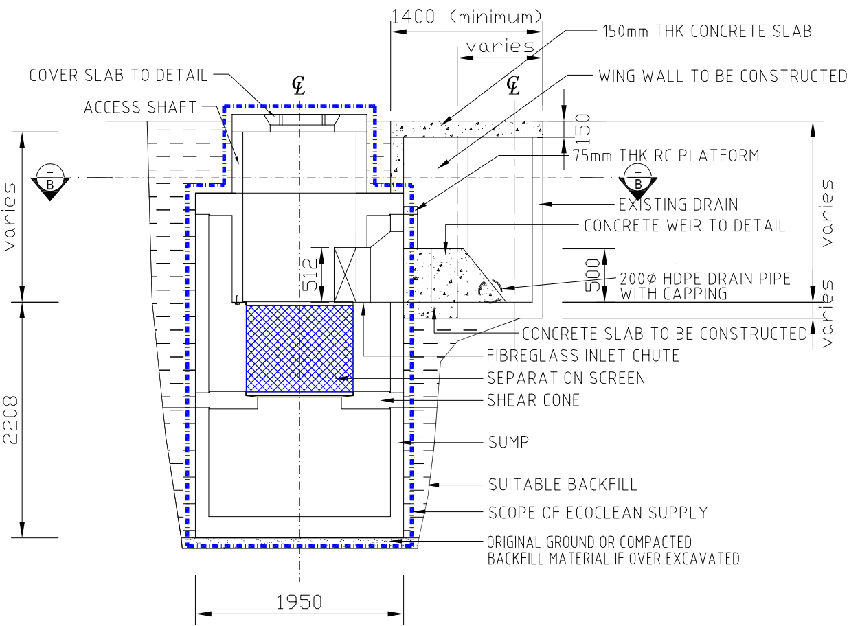
SECTION A-A
