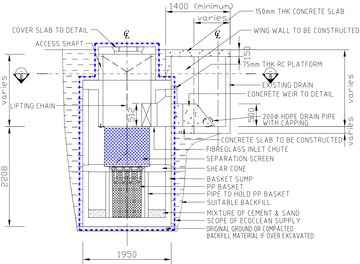
SECTION A-A
