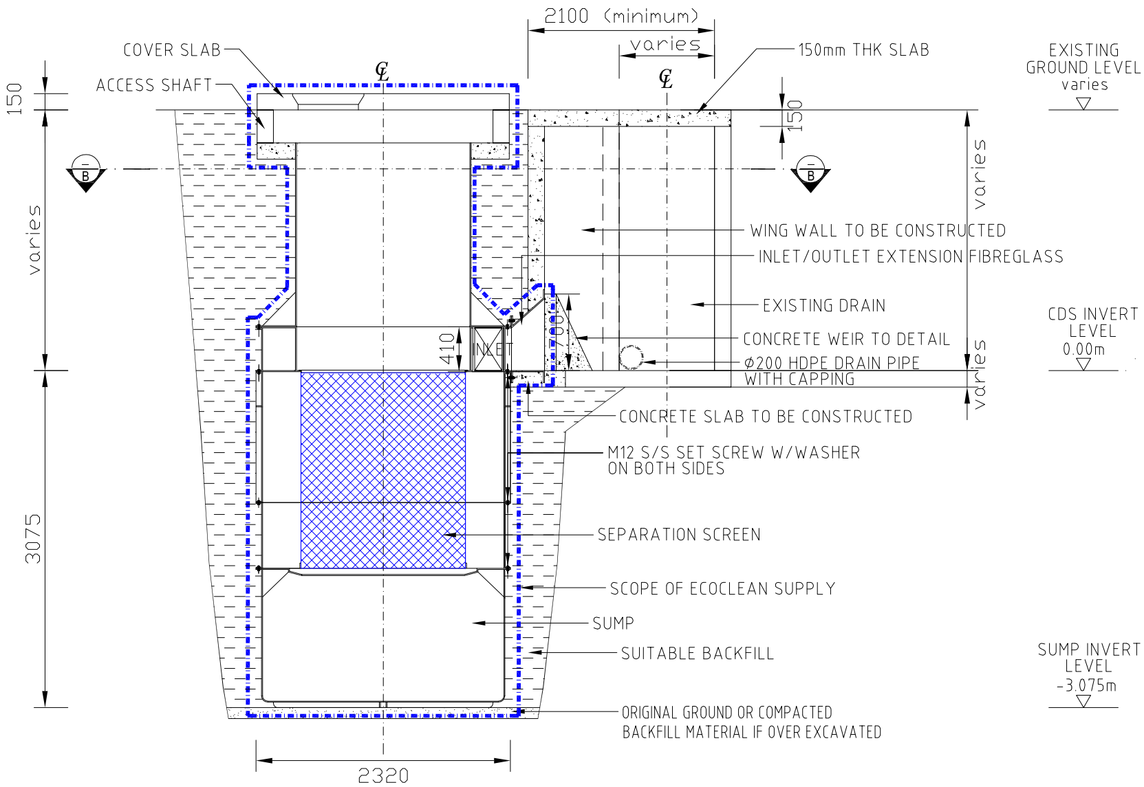
SECTION A-A
