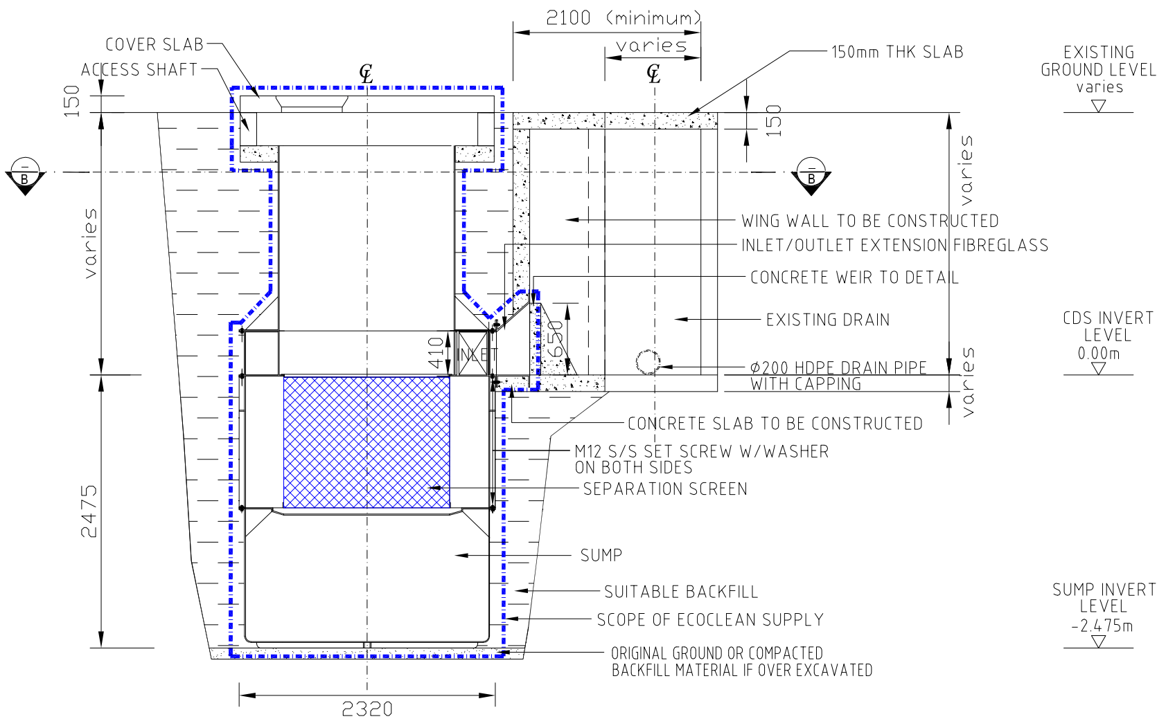
SECTION A-A
