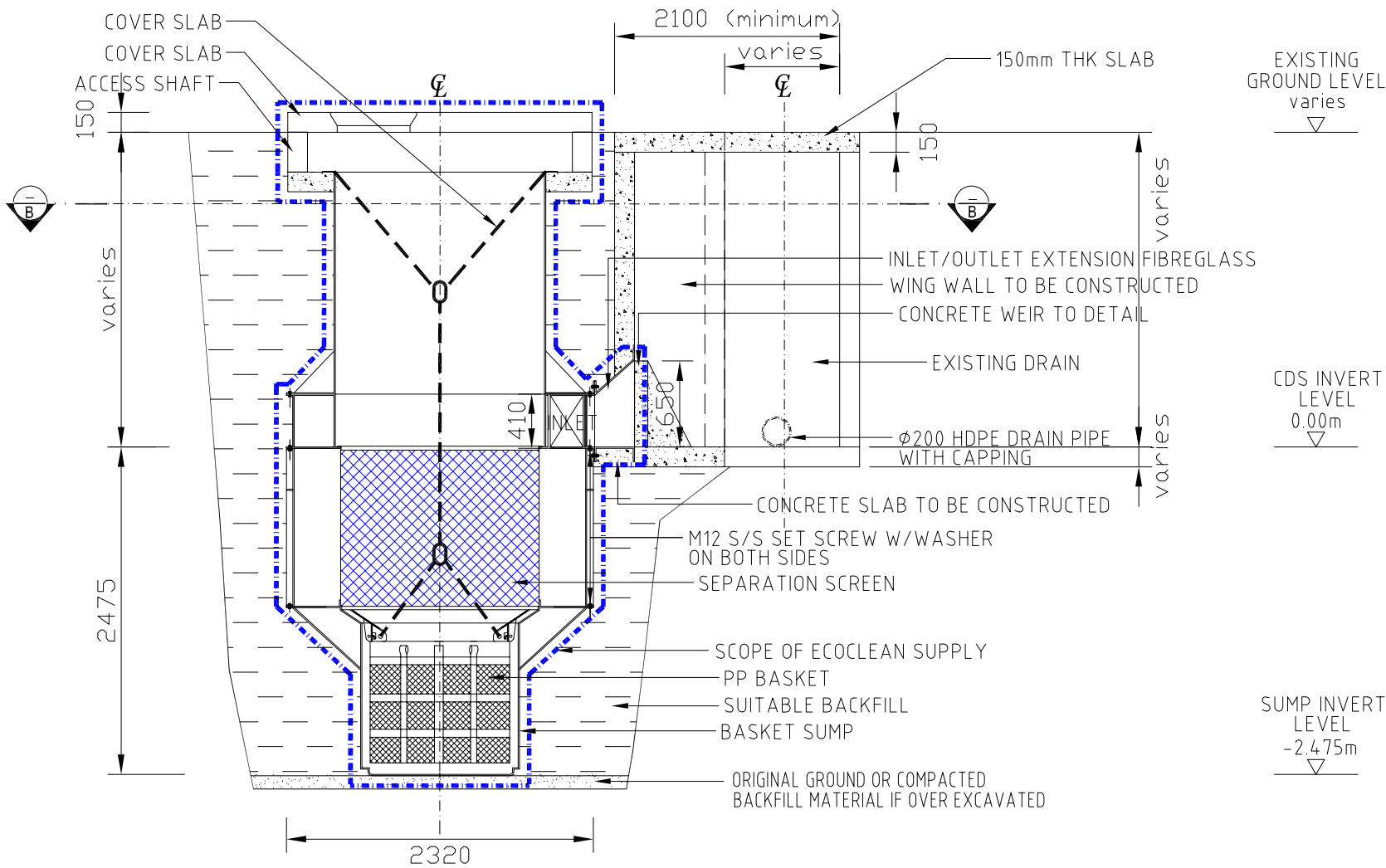
SECTION A-A
