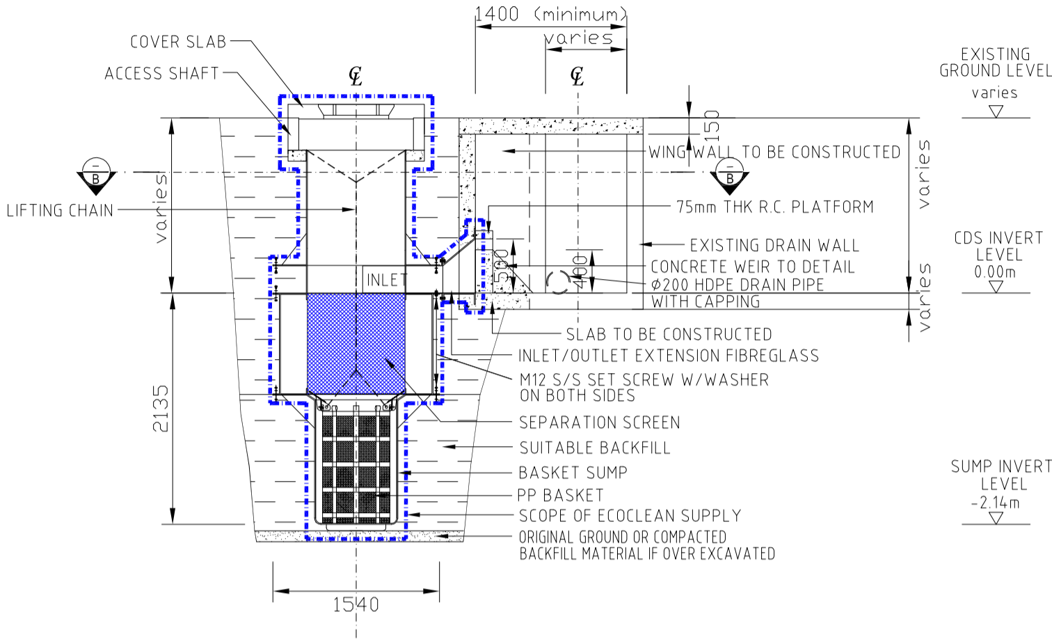
SECTION A-A
